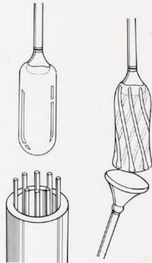
Einbringung des farblosen Glases in die Eisenform und Anschmelzen der Milchglasstäbe
