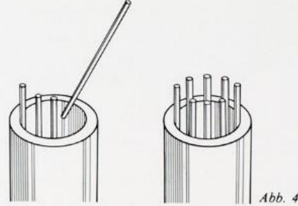
Einordnen von Milchglasstäben in eine Eisenform
